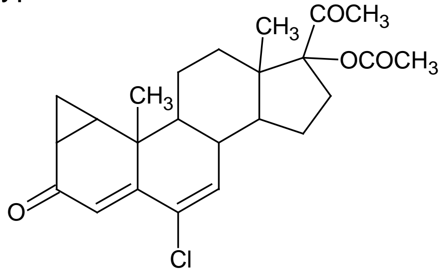
cyproteron acetát
