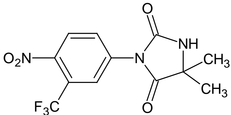
Nilutamid
